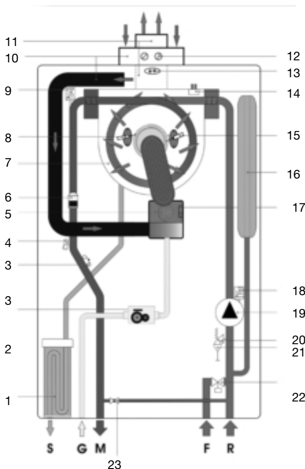
fig. 5 - Schema idraulico modello KR
